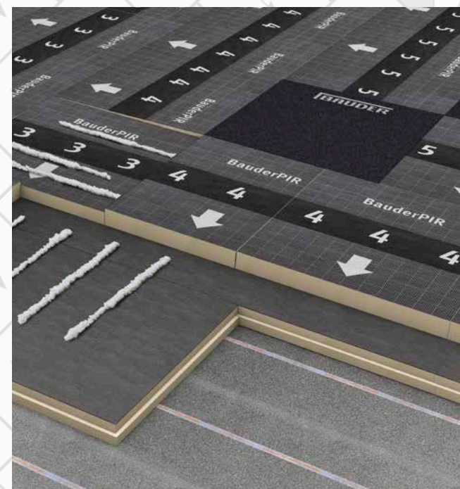
Abb. 6/2: Verlegebeispiel BauderPIR GFS Gratfüllstück
