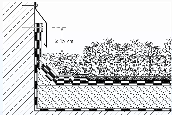
Abb. 2*: Bei Wandanschlüssen fordern die Flachdachrichtlinien bei Dachneigungen bis 5° mind. 15 cm und bei Dachneigungen über 5° mind. 10 cm Anschlusshöhe über Oberfläche Belag oder Kiesschüttung.
