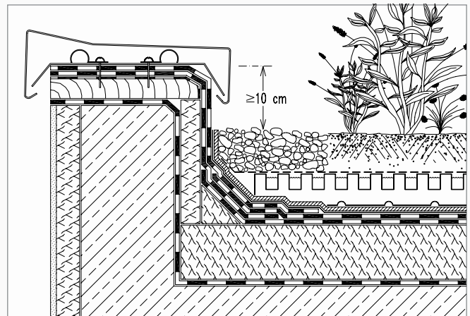
Abb. 1*: Über Oberfläche Belag oder Kiesschüttung fordern die Flachdachrichtlinien bei Dachneigungen bis 5° mind. 10 cm, bei Dachneigungen über 5° mind. 5 cm Höhe des Dachrands.
